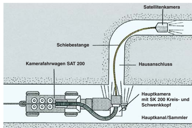
Satellitenkamarasystem
