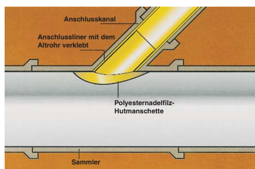
Renovierung im Anschlussbereich des städtischen Kanals
